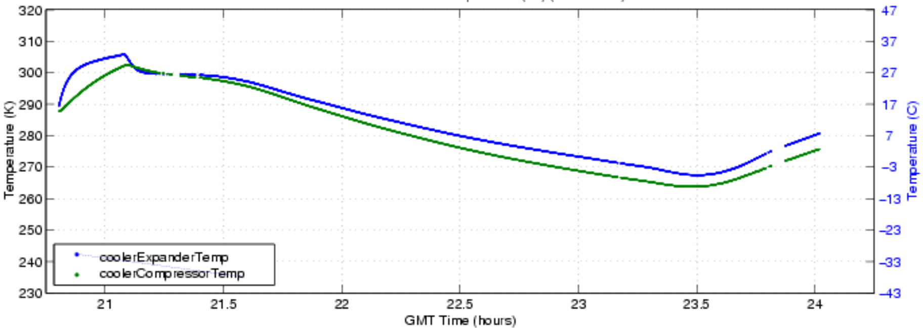
S-HIS Detector Parameters, 041015 (bf) (ENG Plot 4)
