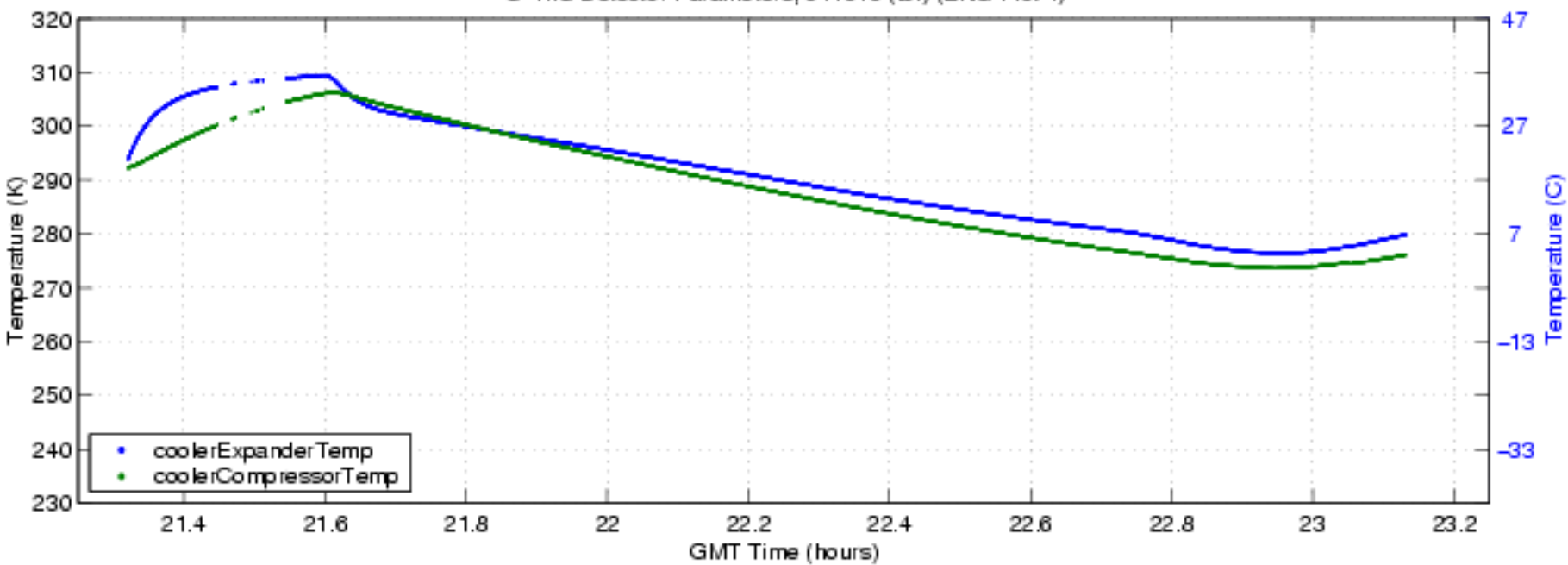
S-HIS Detector Parameters, 041010 (bf) (ENG Plot 4)
