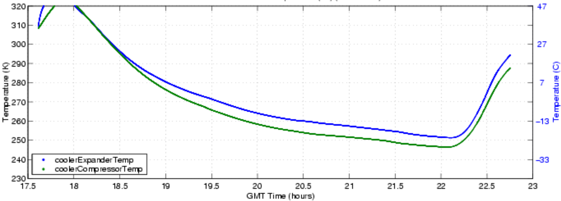
S-HIS Detector Parameters, 050615 (bf) (ENG Plot 5)
