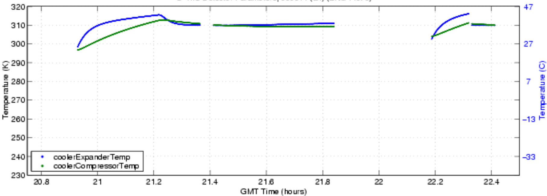
S-HIS Detector Parameters, 050614 (bf) (ENG Plot 5)
