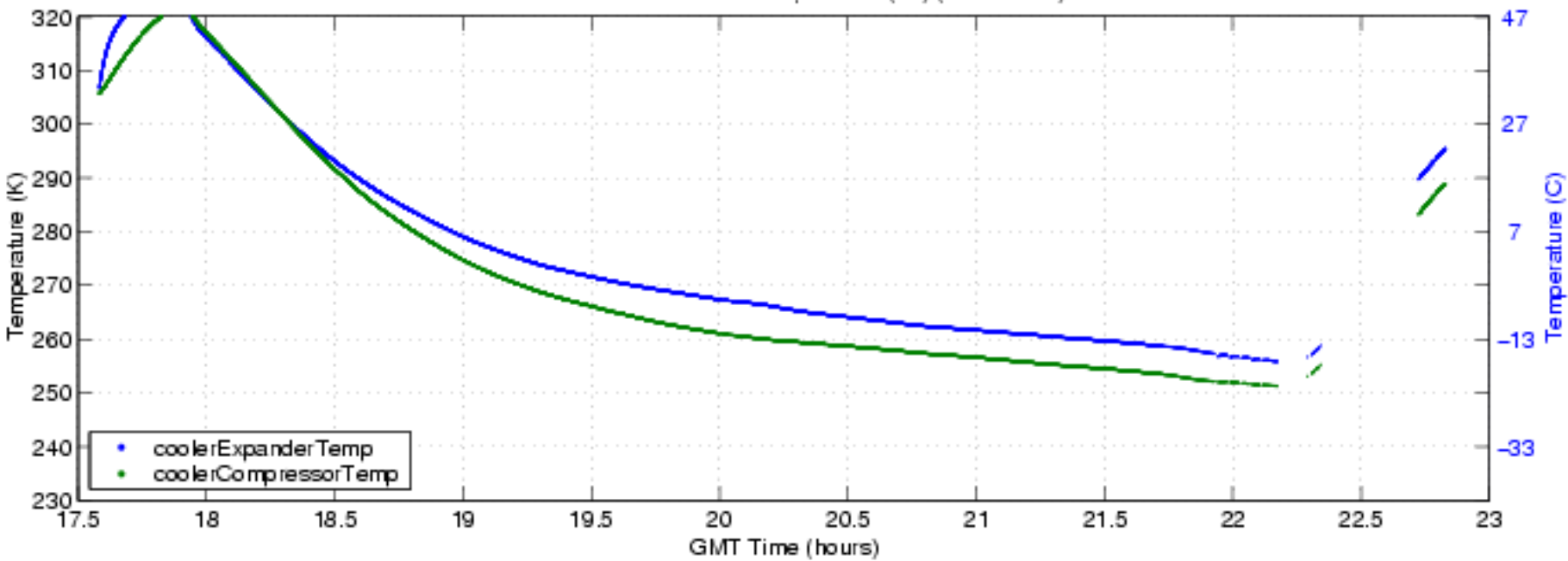
S-HIS Detector Parameters, 050613 (bf) (ENG Plot 5)
